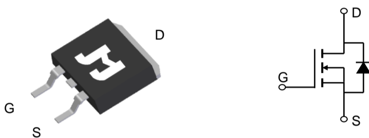
TO-263-3L Top View
