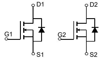
Chip-1 & Chip-2
